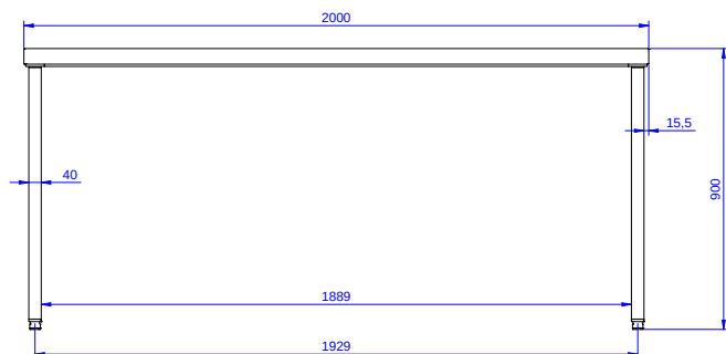
Fronte
